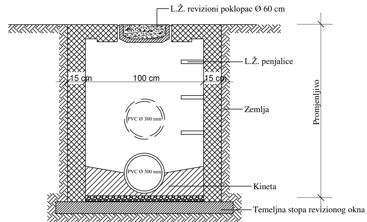
PRESJEK A-A
