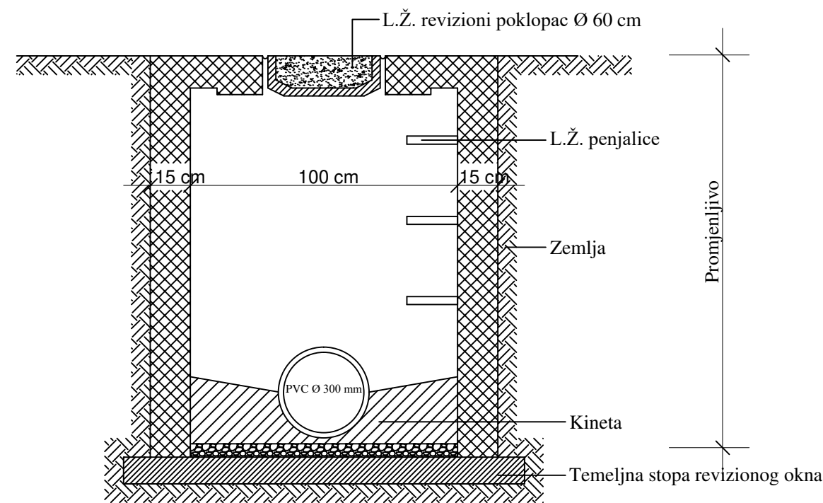
PRESJEK A-A
