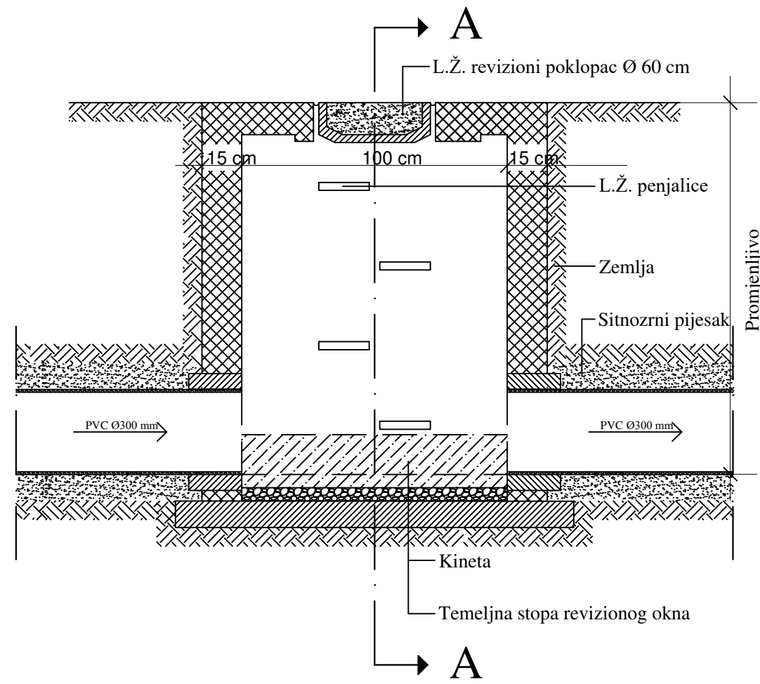
PRESJEK A-A
