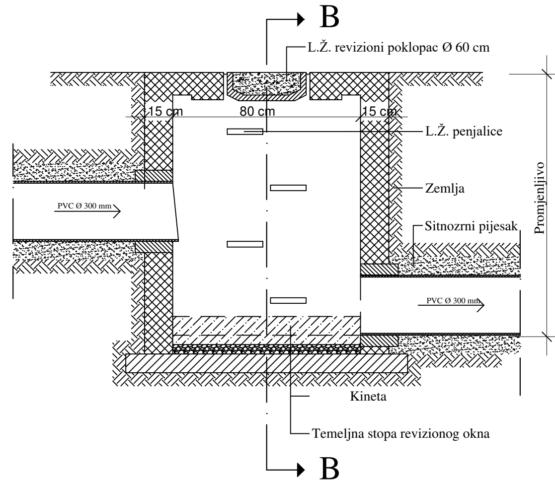
PRESJEK A-A
